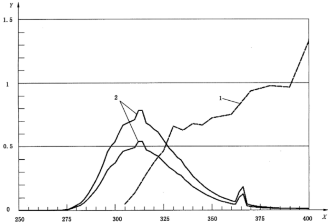
标引说明： X —— 波长( \lambda ),单位为纳米(nm); Y —— 光谱辐照度( E_\lambda ),单位为瓦每平方米纳米[W/(m 2 · nm)]; 1 —— CIE 85:1989 的表 4 中总日辐射; 2 —— 上面的是典型 UVB-313(2 型)灯的光谱辐照度曲线,下面的是 FS40 灯的光谱辐照度曲线。
